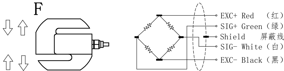
受力示意
