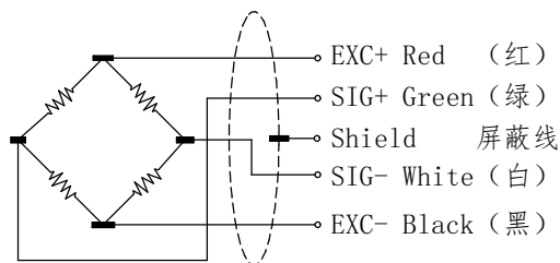
配线图
