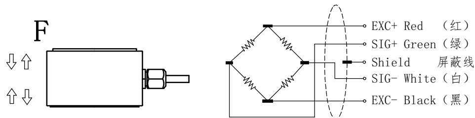
受力示意
