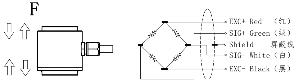
受力示意
